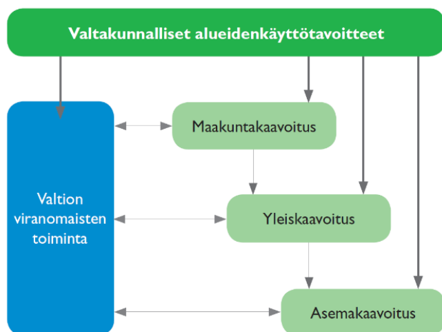
Kuva 9: Kaavahierarkia
