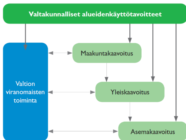
Kuva 7: Kaavahierarkia
